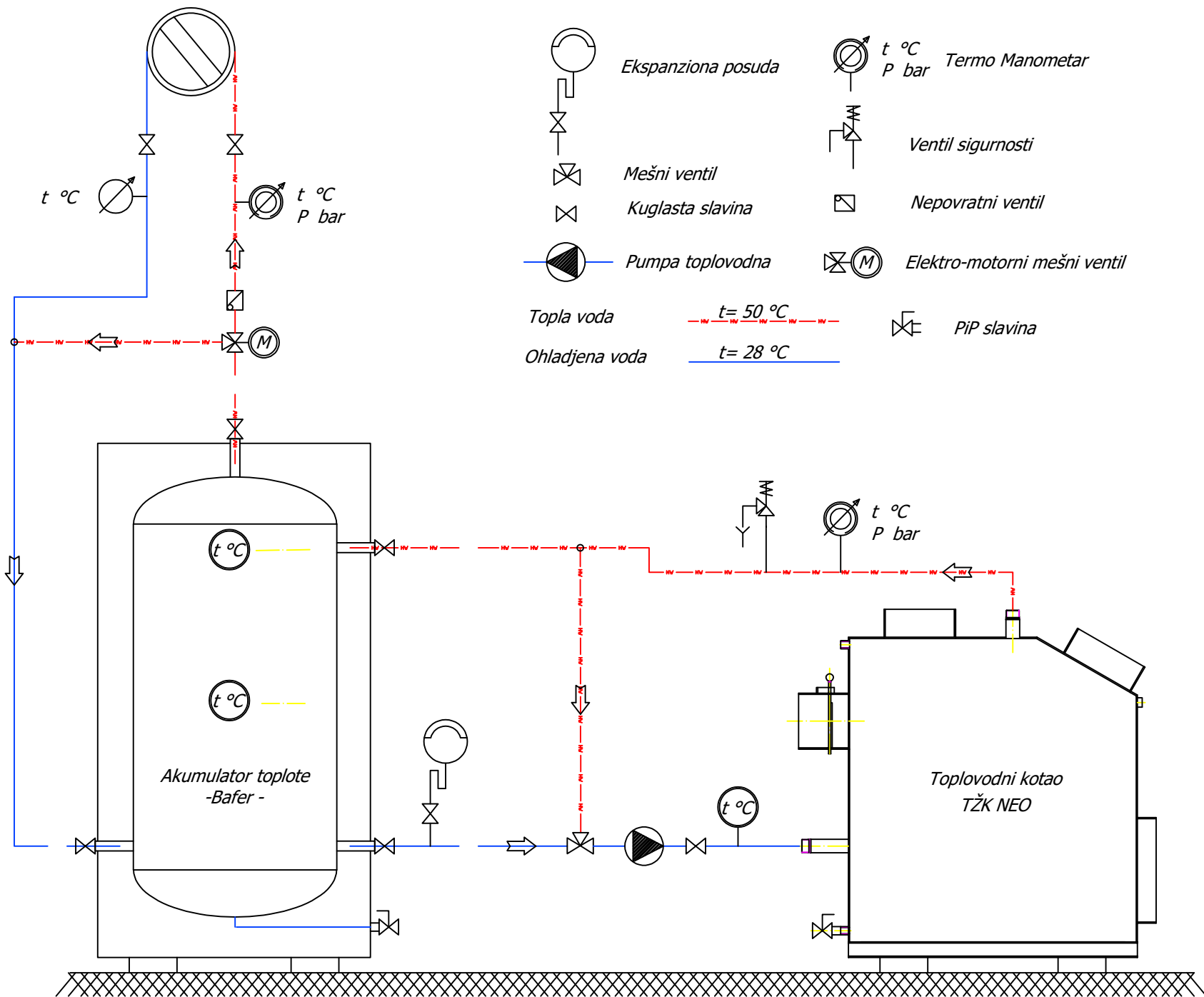
Toplovodni kotao- tehnološka šema povezivanja
